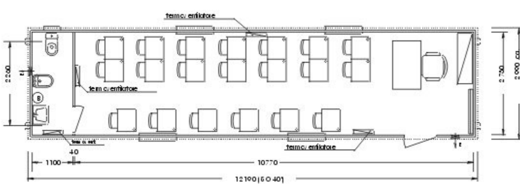
Unità aula scolastica per 20 persone ca.
