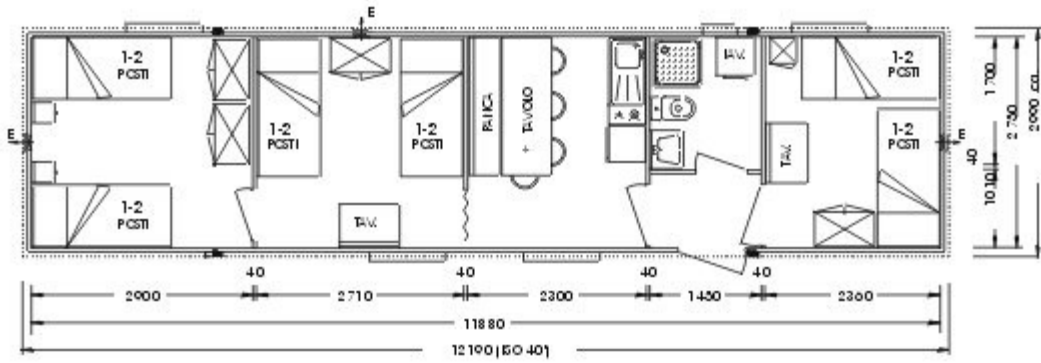
Modulo abitativo per 12 persone (letti a castello)
