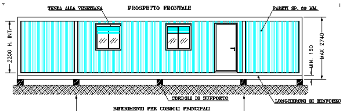
Modulo abitativo di protezione civile tipo m/0/40' unità abitativa per 4 / 8 / 12 persone
