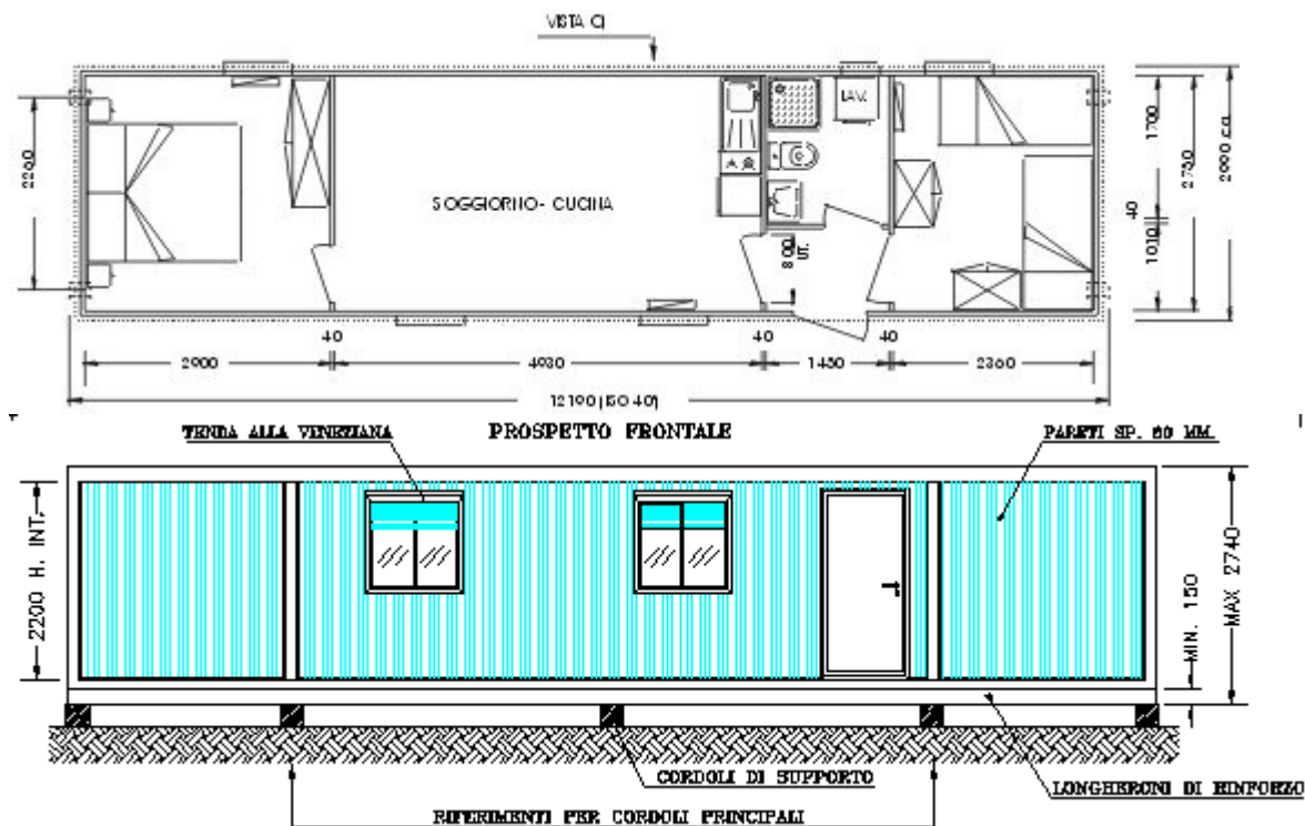
Modulo abitativo arredato
