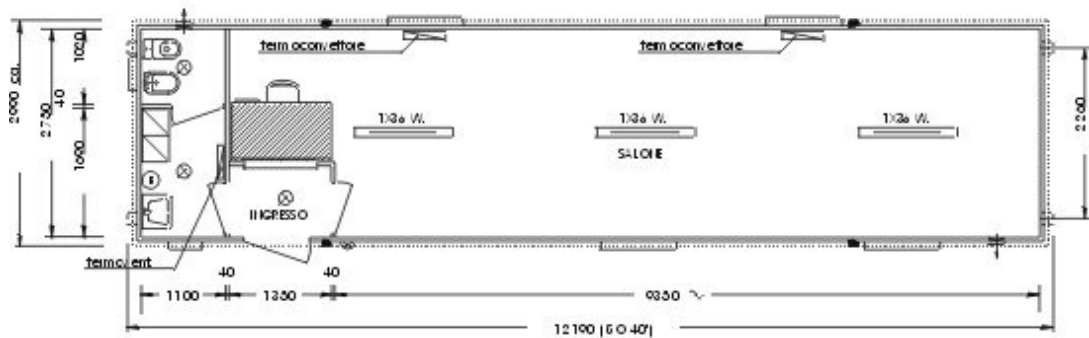
Unità ad uso sociale / ricreativo / Autorità
