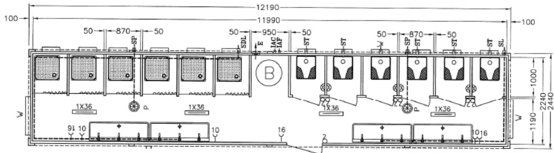
PLANIMETRIA GENERALE (H. INT. MT. 2,70 - EST. MT. 3,00 CA.)
